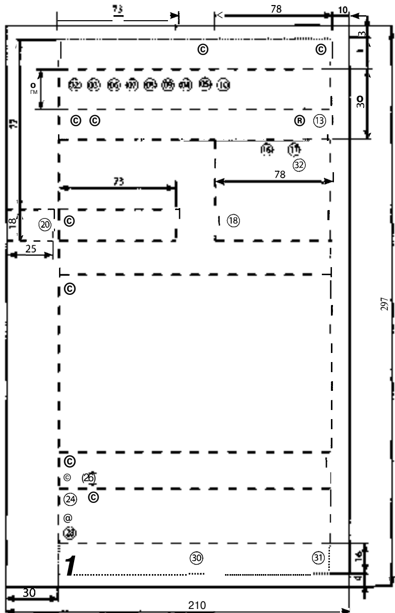
Рис. Б. 1. Розміщення реквізитів і мех зон на форматі A4 поздовжнього бланку
